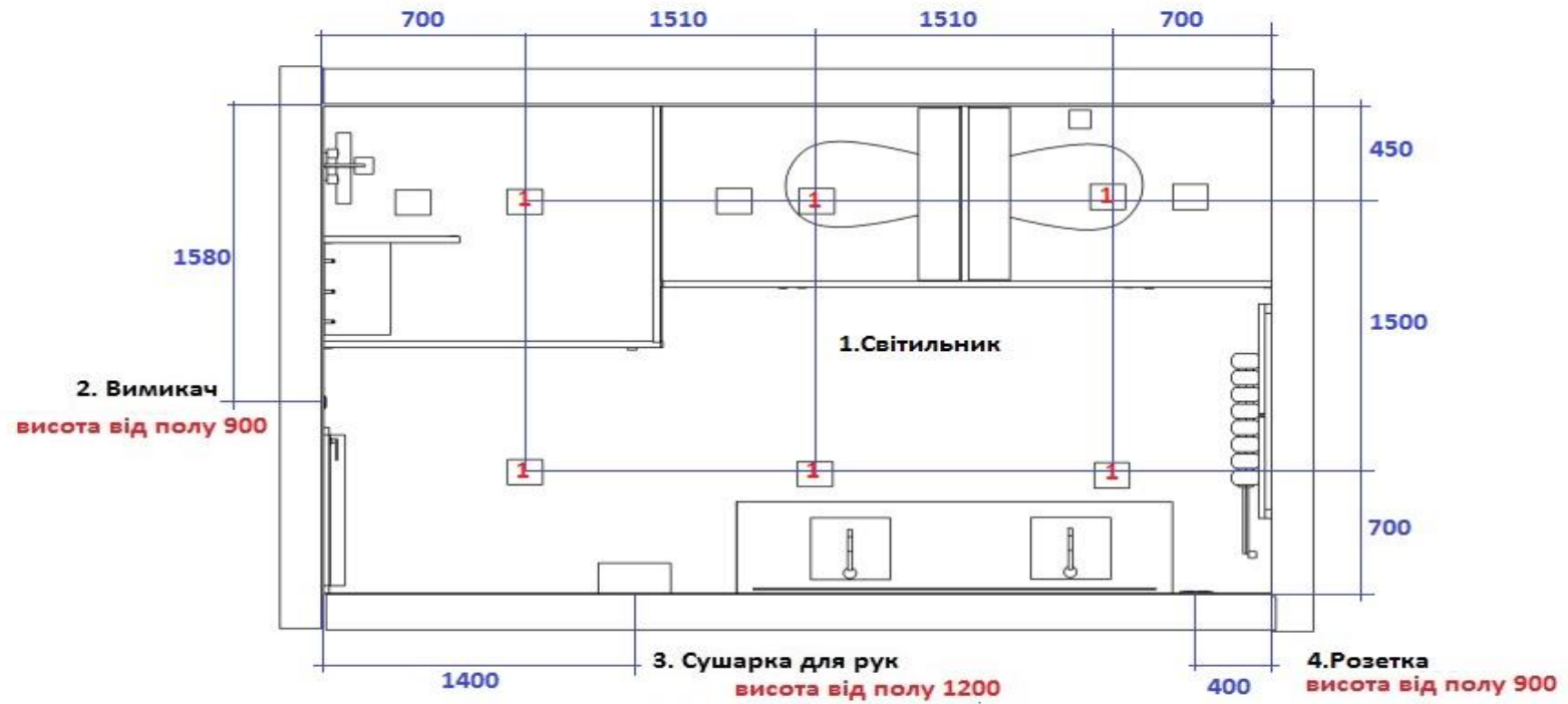
План розташування електричних мереж
